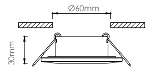
DIMENSIONS
