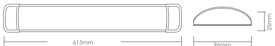
DIMENSIONS
